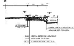
PRZEKROJ "A - A"
