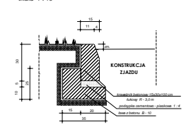
szczegół "C" skala 1 : 10
