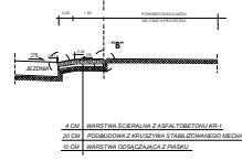
PRZEKROJ "A - A"
