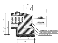
szczegół "A" skala 1 : 10
