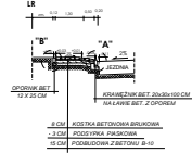
PRZEKROJ "A - A"
